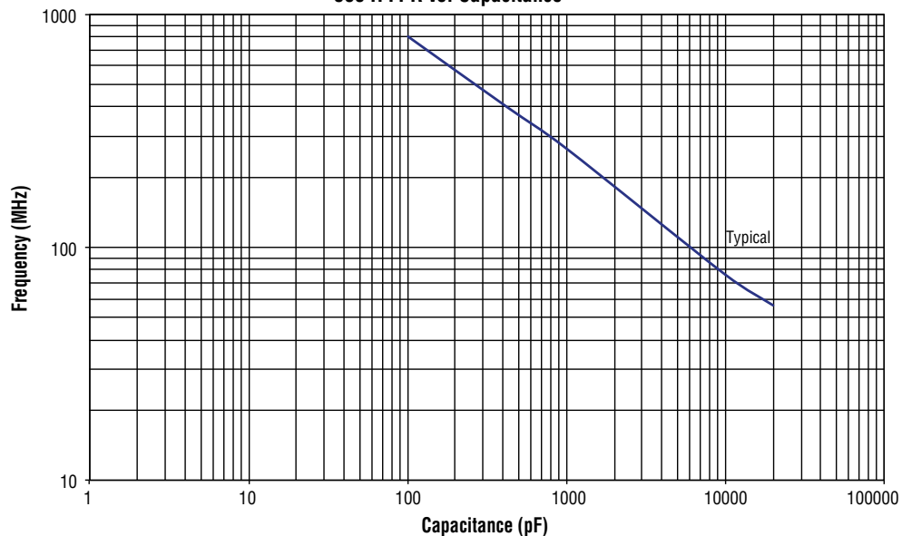
800 H FPR vs. Capacitance
